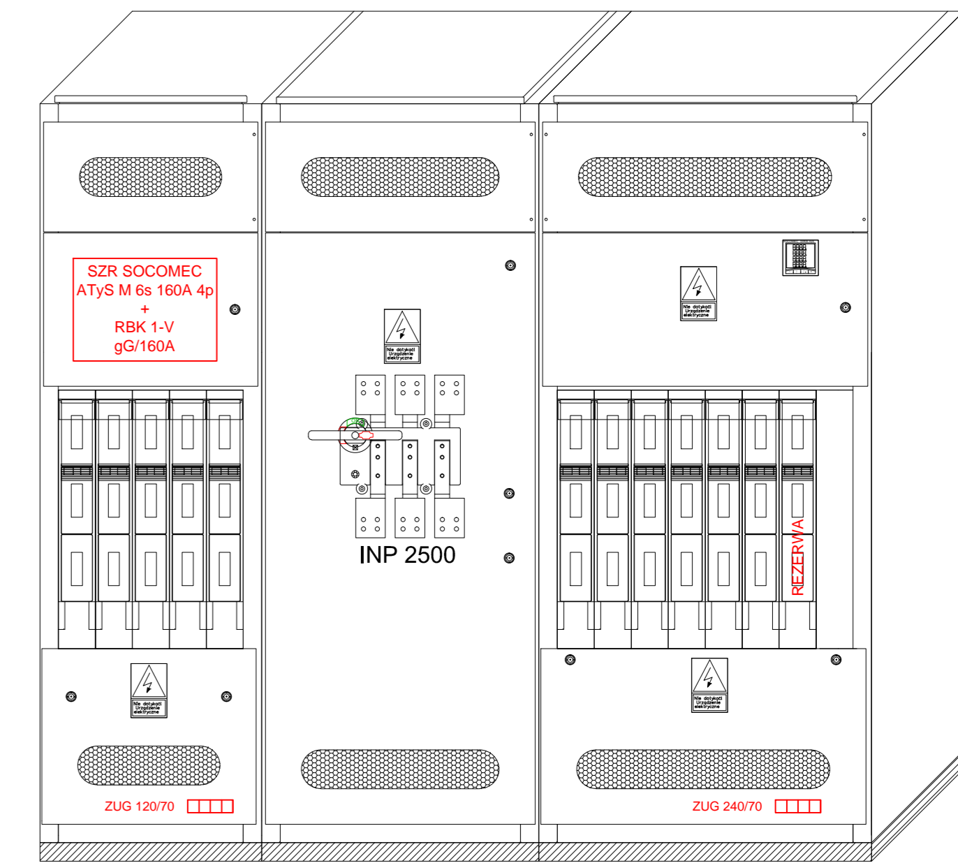
Widok elewacji rozdzielnicy RGnn
